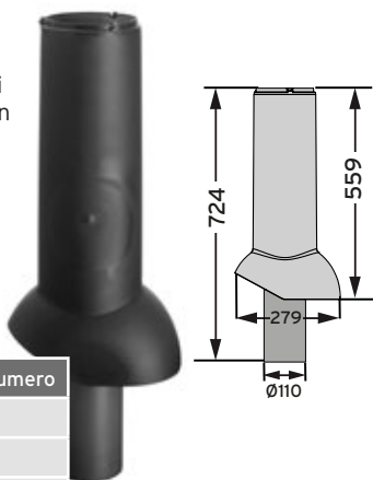
MX-tuuletusputki 110, eristetty
