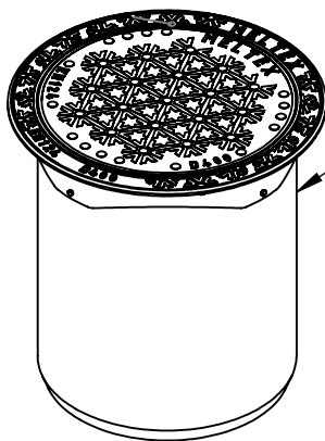
630 mm Teleskooppi
