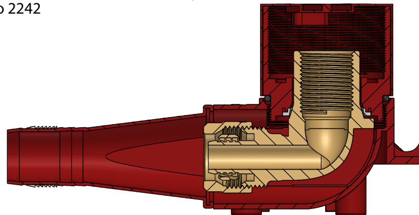
SECTION A-A SCALE 1 : 1.5
