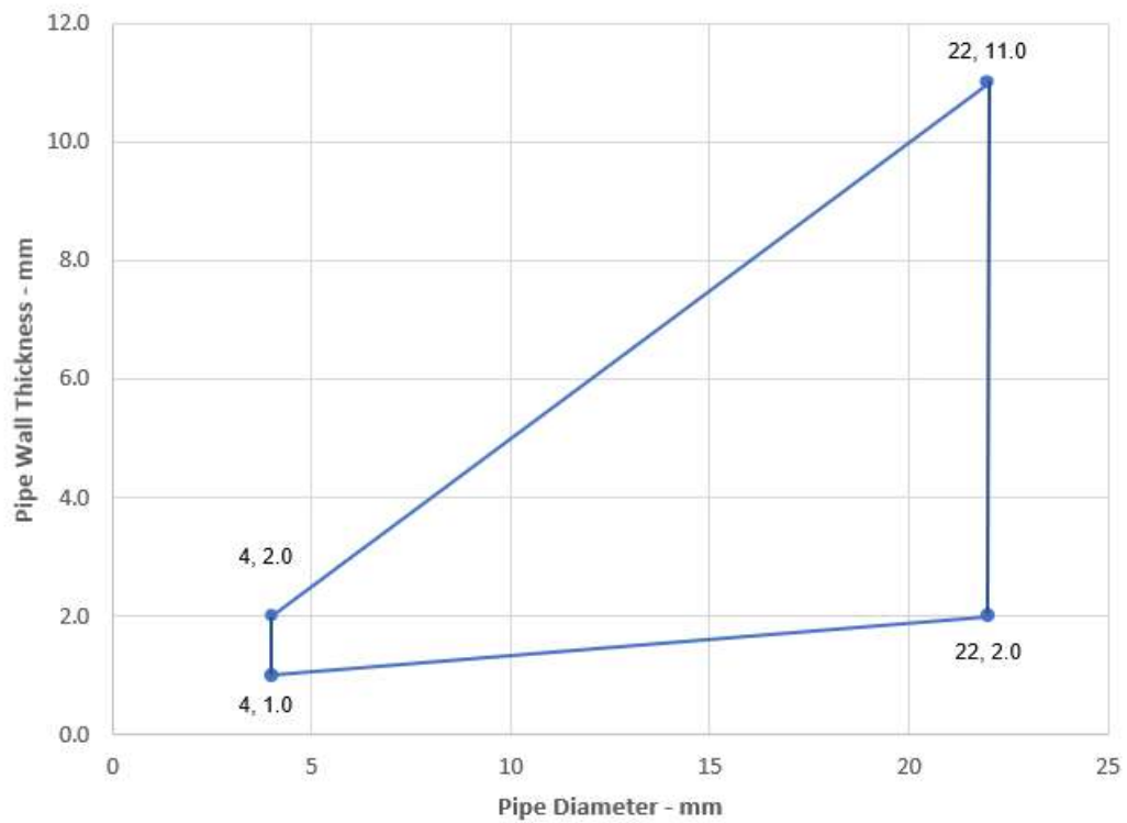
Mild or Stainless Steel Pipes - E 120 C/U, EI 60 C/U
