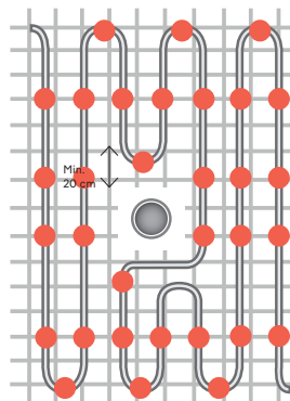
Cable Clip 5
